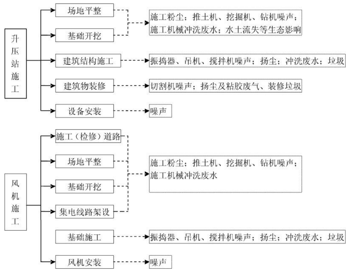
图5-1 施工期工艺流程及产污环节图
