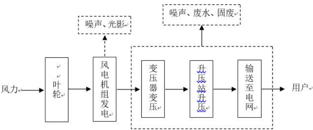
图5-2 风电场运营期工艺流程及产污环节图
