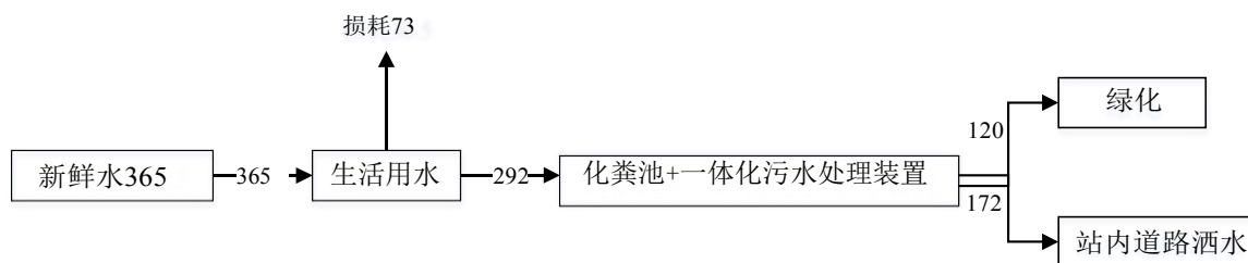
图5-3 建设项目水平衡图 (m³/a)
